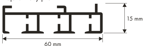
trojdrážkový profil
