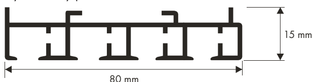
čtyřdrážkový profil
