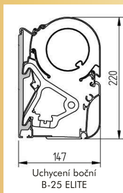
Uchycení boční B-25
