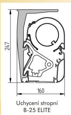
Uchycení stropní B-25
